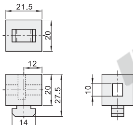
AMV51-308
