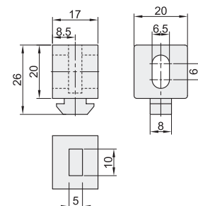
AMV61-308
