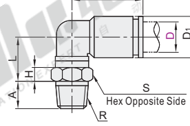
90° Elbow XZC21
