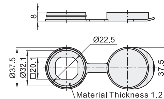
Dust Cap
