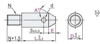
Tapered PAJ71 PAJ76
