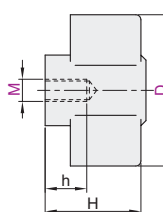
Tapped HAQ16
