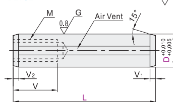
Air Vent, Tolerance +0,010 +0,005 BLV52
