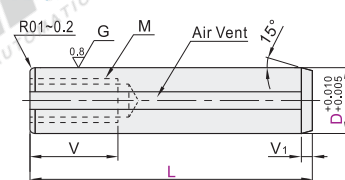
Air Vent, Tolerance +0,010 +0,005 BLV51
