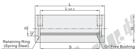
Long Type OGX22
