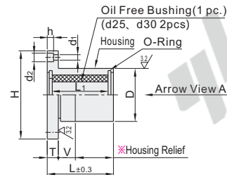
Round Flange OFZ81
