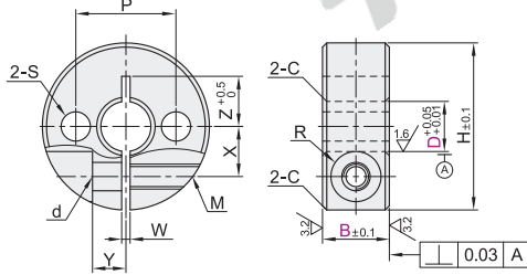
2-Hole FAJ01/02/06
