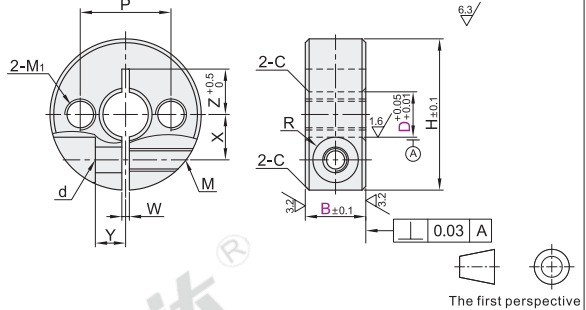
2-Tapped FAJ51/52/56
